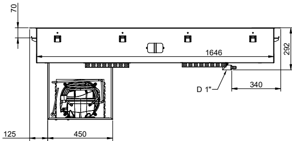
Zij aanzicht
